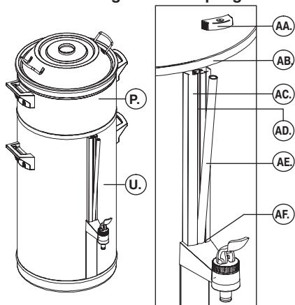
Fig. 8 Reinigen van het peilglas
